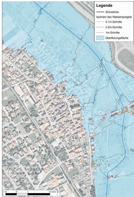
Gegenwart und Zukunft: Das linke Bild zeigt die Überschwemmungssituation in Dittigheim bei einem 100-jährigen Hochwasser, wie sie sich zurzeit darstellt. Das rechte Bild zeigt die Situation, wie sie nach der Realisierung der Hochwasserschutzmaßnahmen sein wird. Die roten Linien markieren den Damm, der bis zu 2,80 Meter hoch wird, die dünne schwarze Linie stellt die Spundwand dar.
